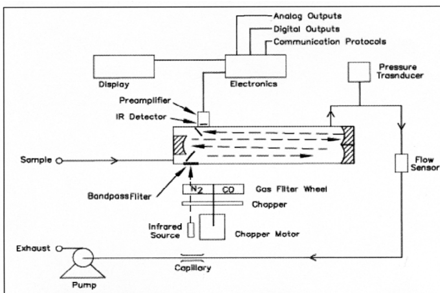
Figur 1: Principskiss för instrumentet Carbon Monoxide Analyser CO12M.
